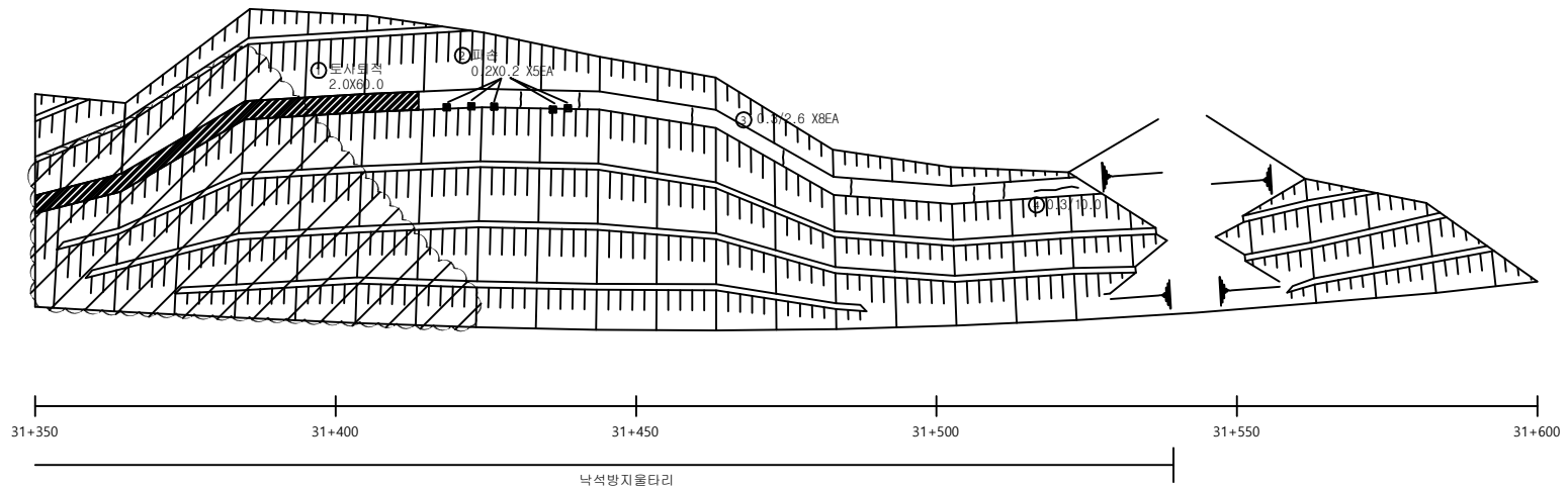
절토사면 / 관리이정 STA.31+100~31+600(좌)
